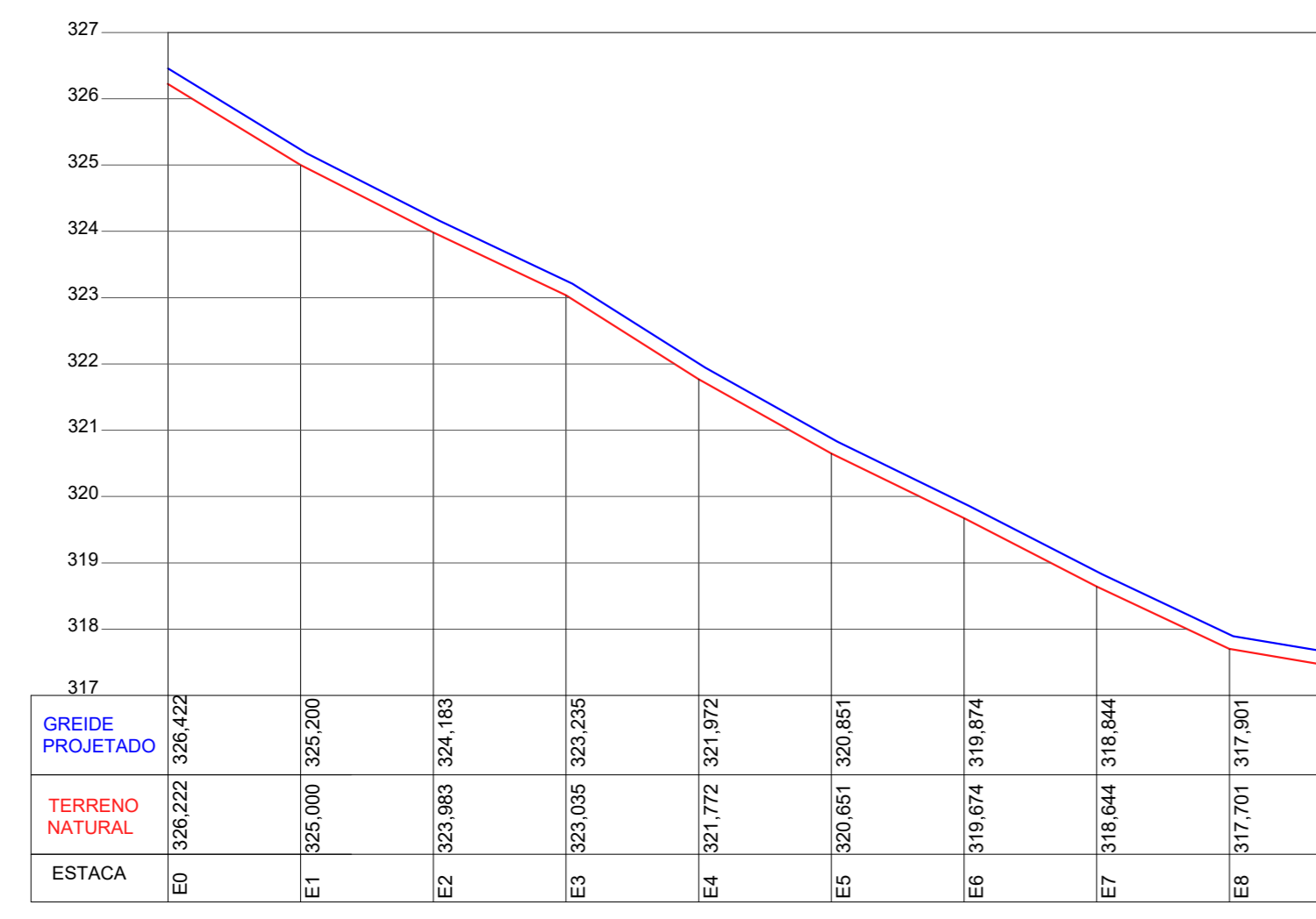
PERFIL LONGITUDINAL EIXO DA RUA FRANCISCO DE ASSIS DA SILVA ESCALA H 1/1000 V 1/100
