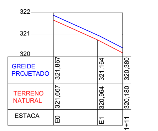
PERFIL LONGITUDINAL EIXO DA TRAVESSA 08 ESCALA H 1/1000 V 1/100
